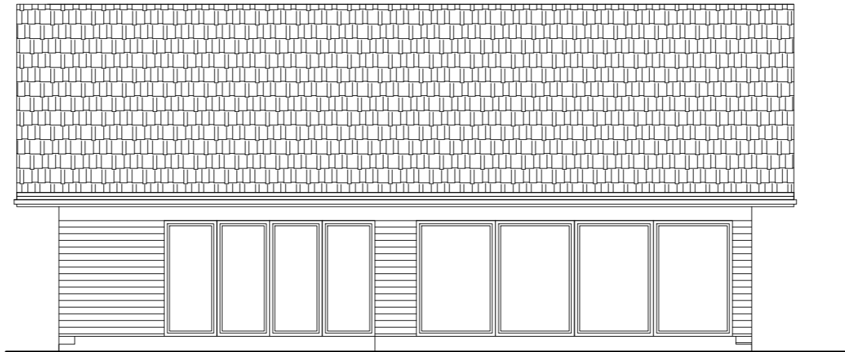
ELEWACJA OGRODOWA
